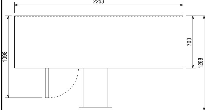
Boven aanzicht
